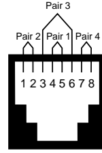
T568B
