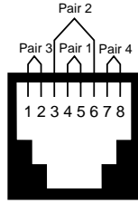
T568A
