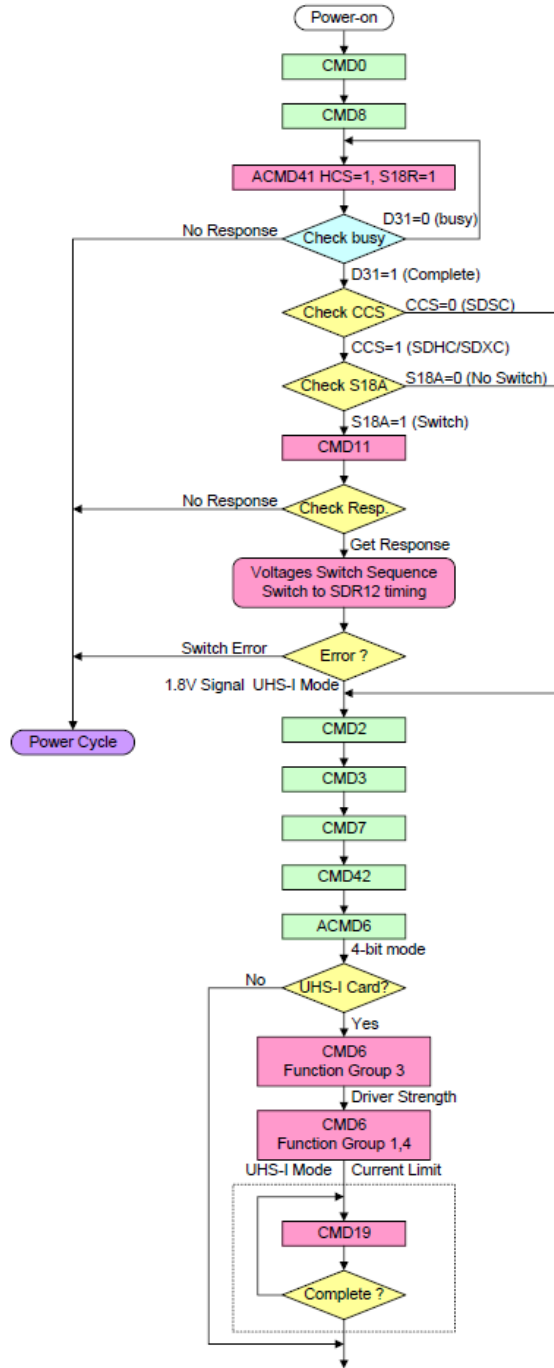
Şekil 4-1: UHS-I Ana Sistem Başlatma Akış Şeması
