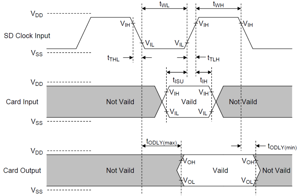
Şekil 6-1: AC Zamanlama Şeması (Varsayılan)
