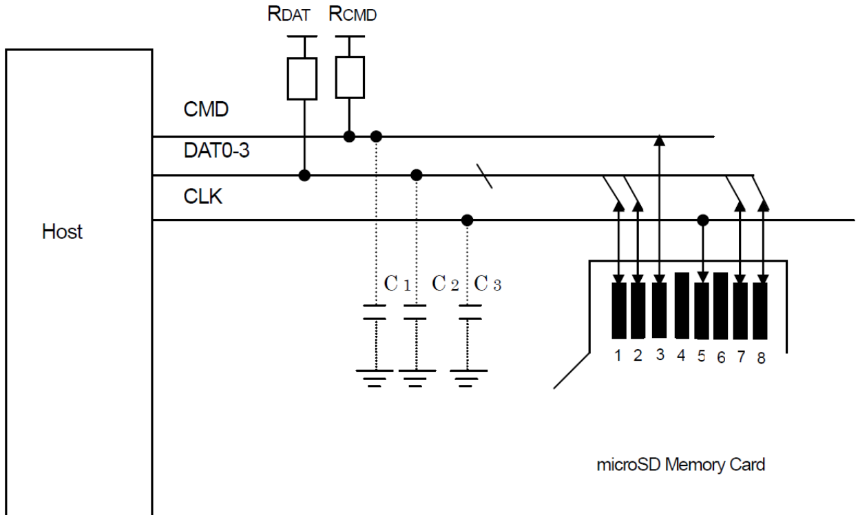
Şekil 5: microSD Kart Bağlantı Şeması
