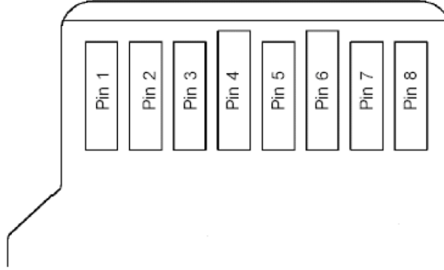
Şekil 1: microSD Kart Pim Atamaları (Kartın Arkadan Görünümü)
